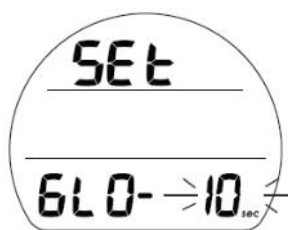
Fig. 33 - SET GLO
