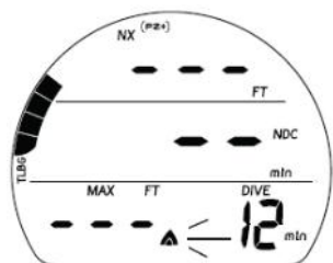
Fig. 69 - DV 3 MAIN
